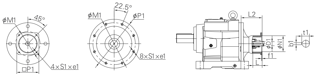
AS040-AS315
